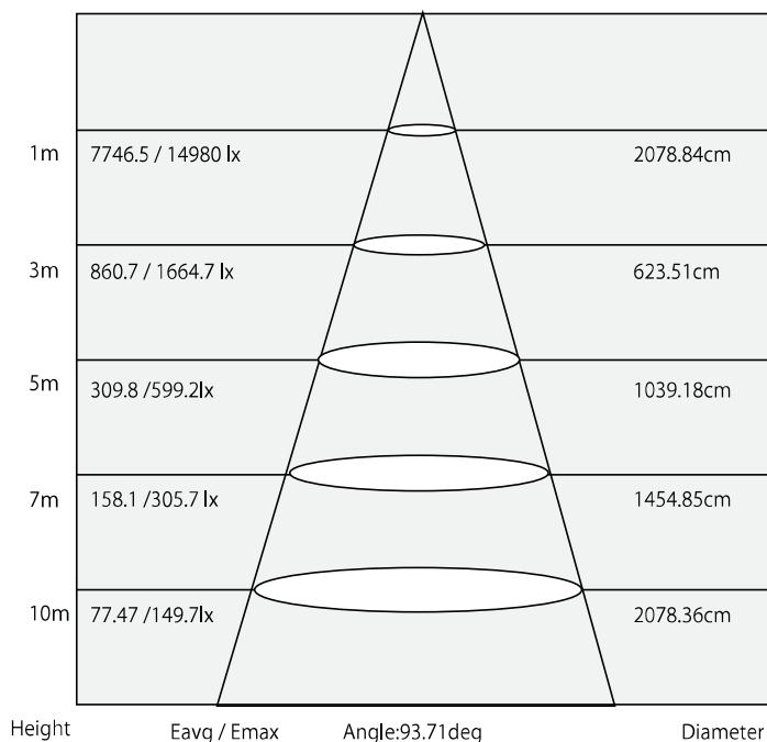
配光表
