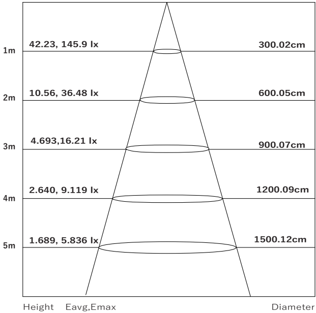
直下照度分布図
